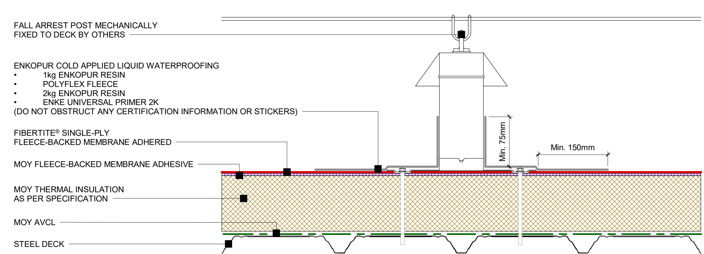
17 FiberTite® - Fall arrest detail (Enke) 1 : 5
