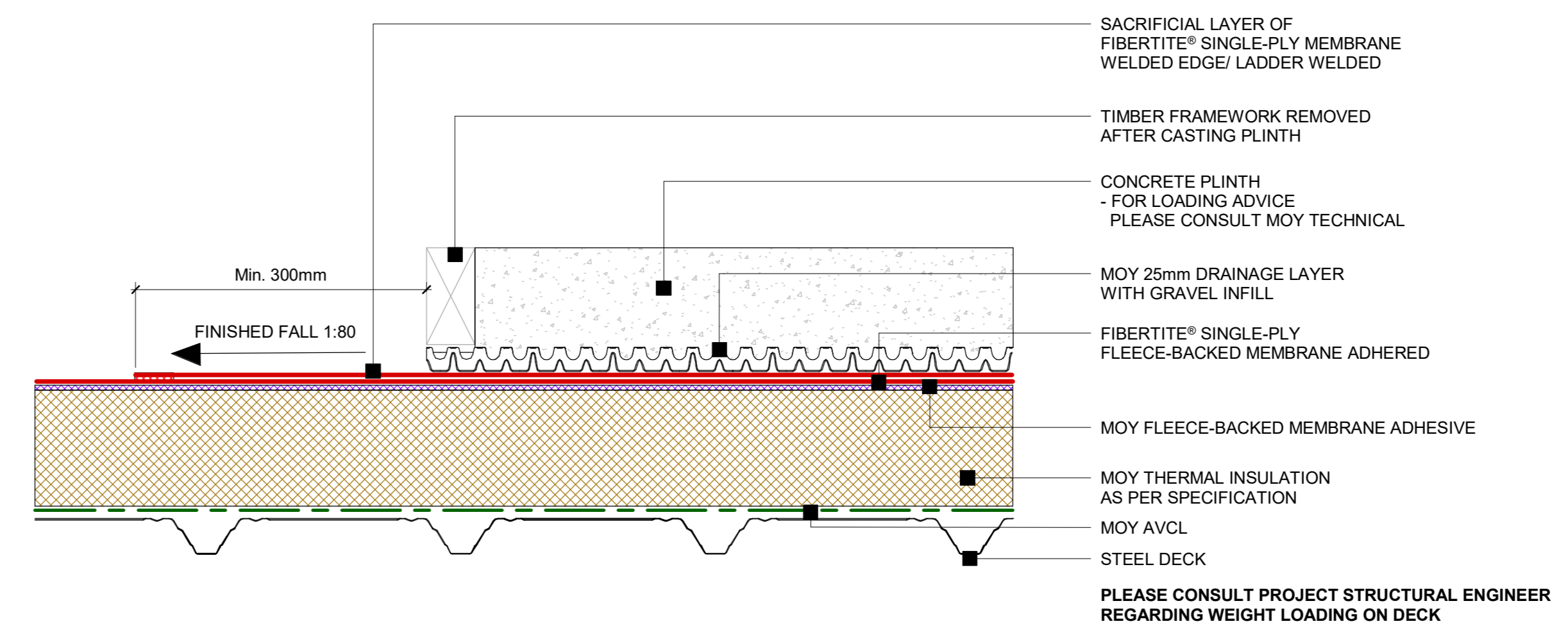
26 FiberTite® - Poured concrete plinth detail 1 : 5
