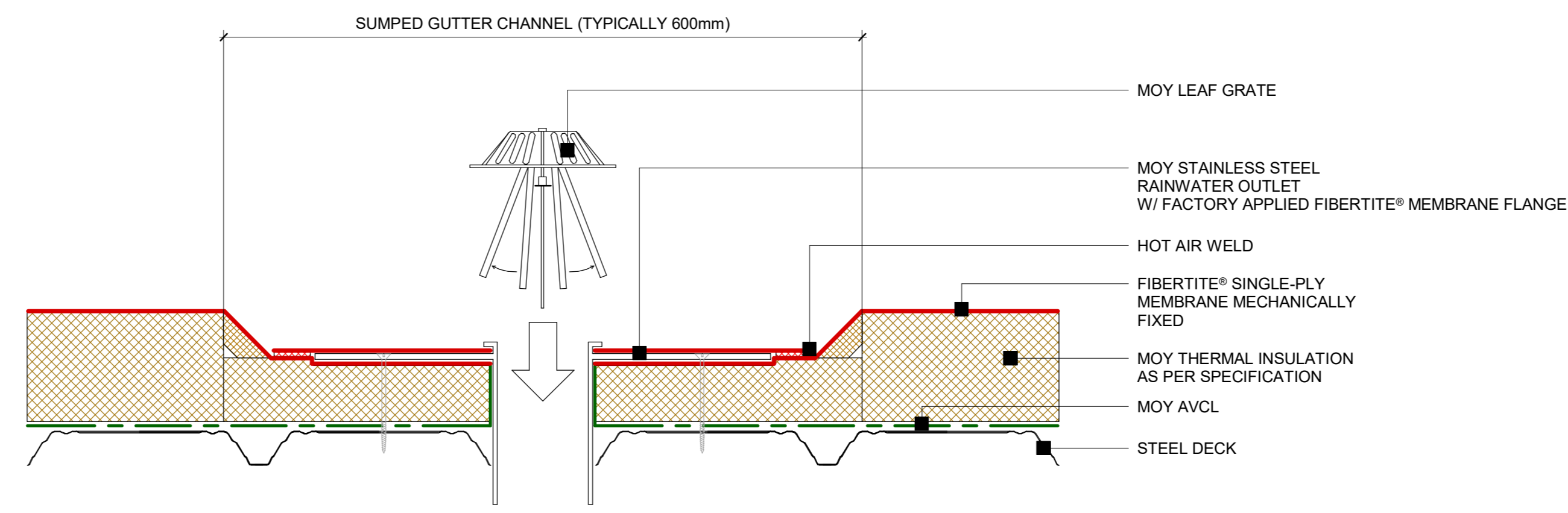
5 Fibertite® - Rainwater outlet detail 1 : 5
