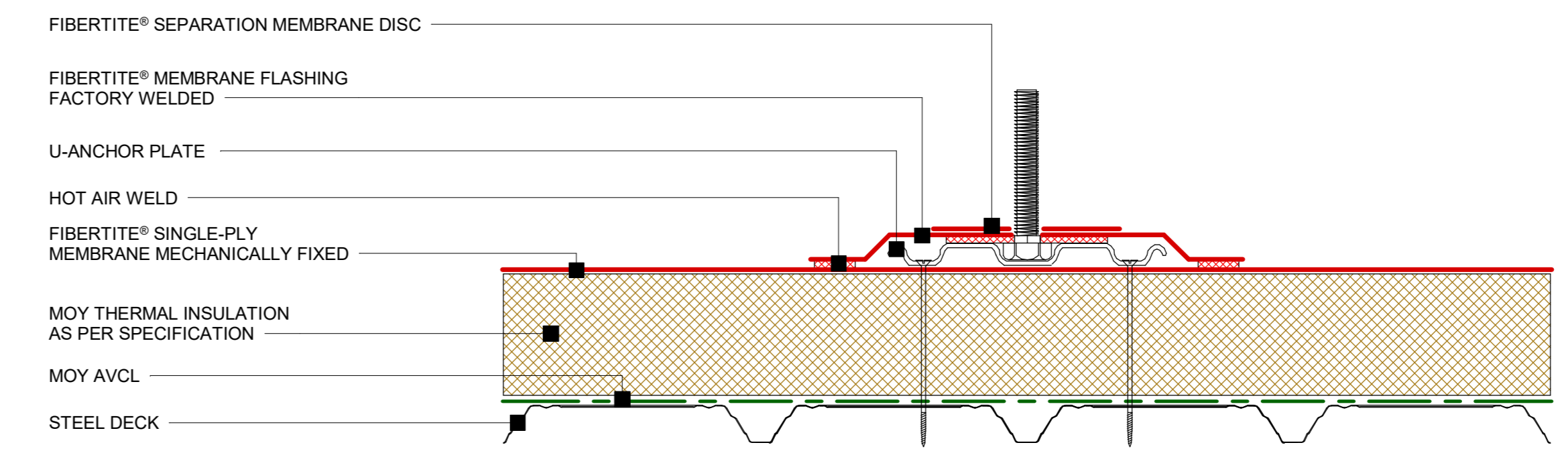
20 FiberTite® - U Anchor detail 1 : 5
