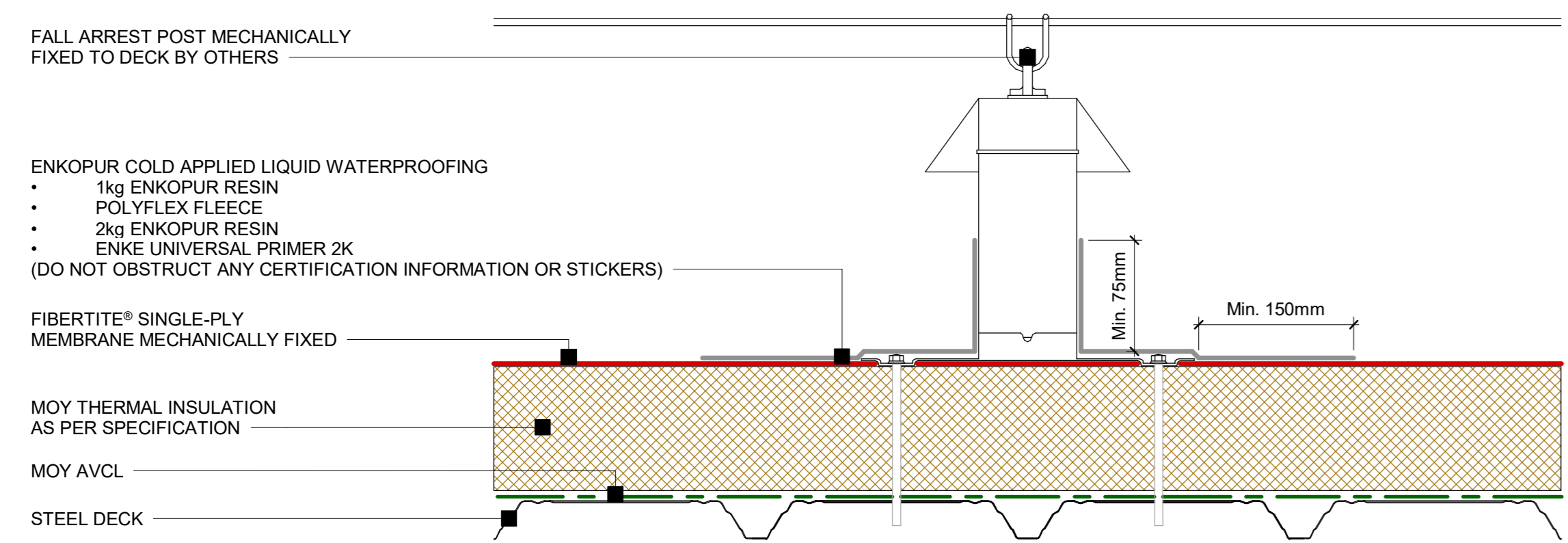
17 FiberTite® - Fall arrest detail (Enke) 1 : 5
