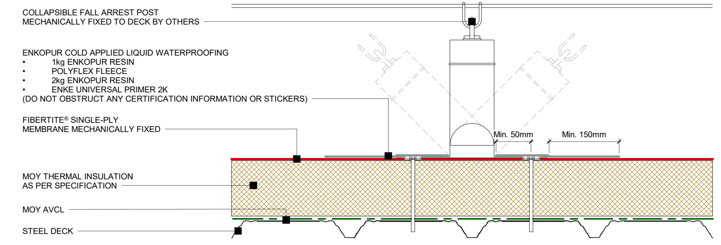
18 FiberTite® - Collapsible fall arrest detail (Enke) 1 : 5
